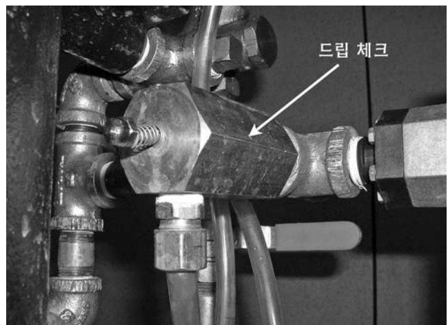
29. 중간 밸브 챔버에서 새는 곳이 없는지 확인하십시오. 알람 라인의 드립 체크는 물 또는 에어를 누출해서는 안 됩니다.
