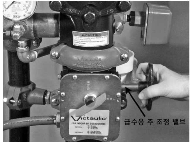
5. 급수용 주 배수 밸브를 통해 물이 적은 양이라도 흘러나올 때까지 급수용 주 조정 밸브를 천천히 여십시오.
