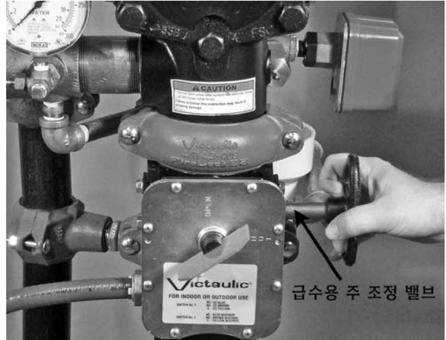
27. 물이 열려있는 급수용 주 배수구 밸브로부터 꾸준히 흘러나올 때까지 급수용 주 조정 밸브를 여십시오.
