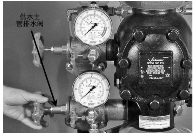
28. 물이 꾸준히 흘러나오면, 급수용 주 배수 밸브를 닫으십시오.
