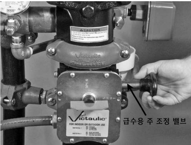
5. 급수용 주 조정 밸브를 닫으십시오.
