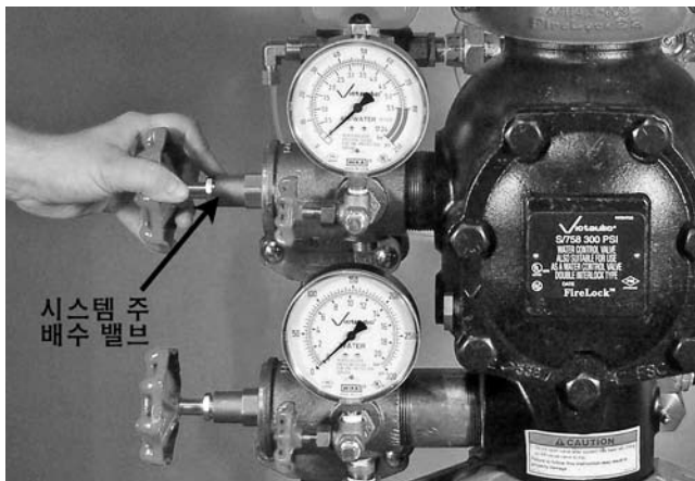
2. 시스템의 주 배수 밸브를 닫으십시오.
