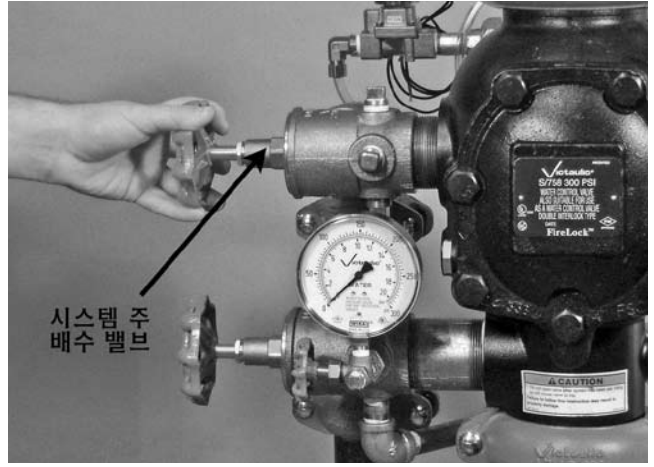
8. 시스템 주 배수 밸브를 닫으십시오.
