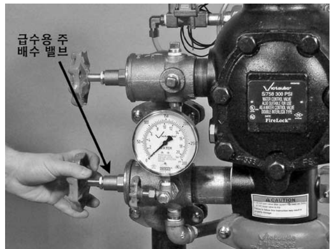
6. 급수용 주 배수 밸브를 닫으십시오.
