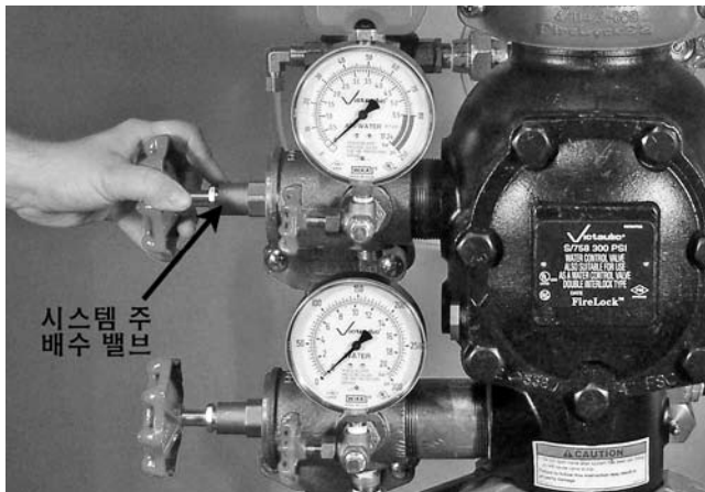
1. 시스템의 주 배수 밸브를 여십시오. 시스템의 배수 상태를 확인하십시오.
