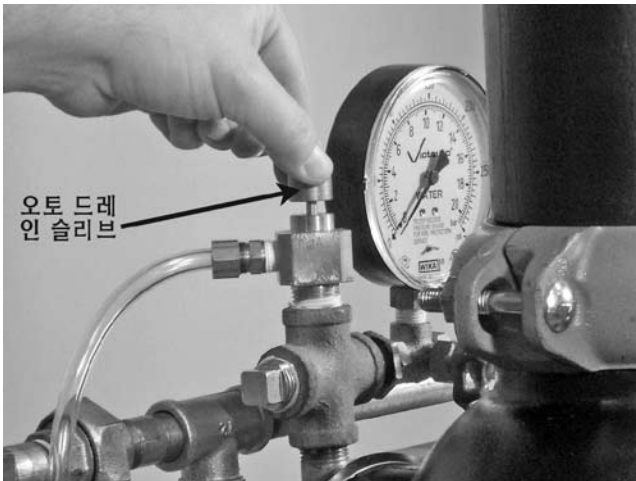
21. 스크류가 위로 향하는 위치에 이를 때까지 오토 드레인의 슬리브를 위로 올리십시오. 다이어프램 압력전달관으로 가는 압력이 있는지 게이지를 통해 확인하십시오.
