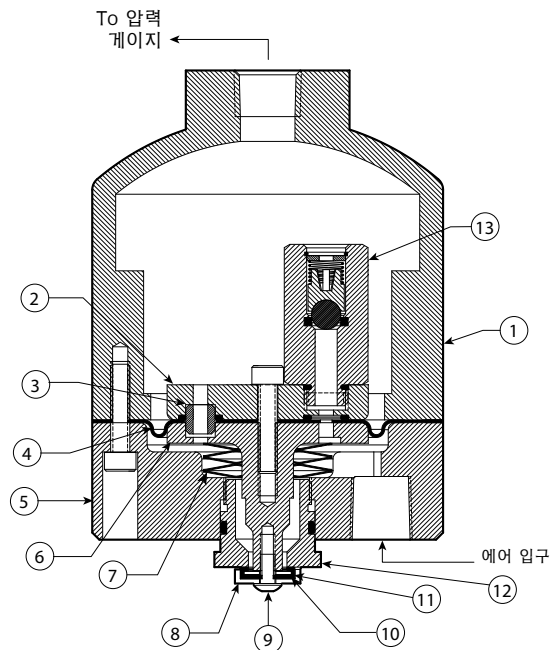
단면도 (선명도를 위해 볼트 부분 제거, 상단 챔버 45도 회전시켰음)
